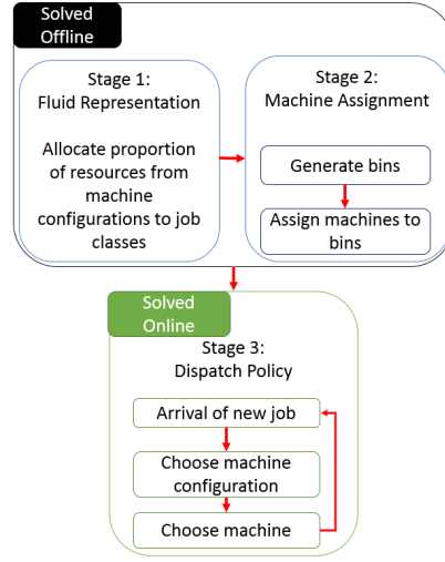
Fig. 4: LoTES Algorithm.
